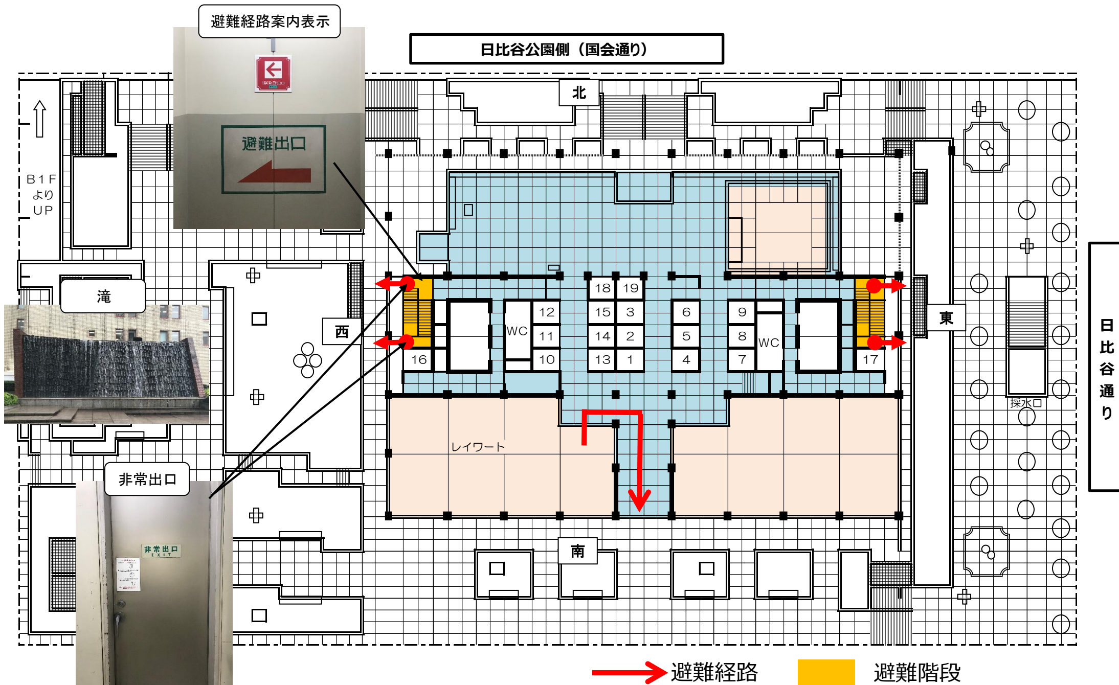
別図5 避難経路 (1F)
