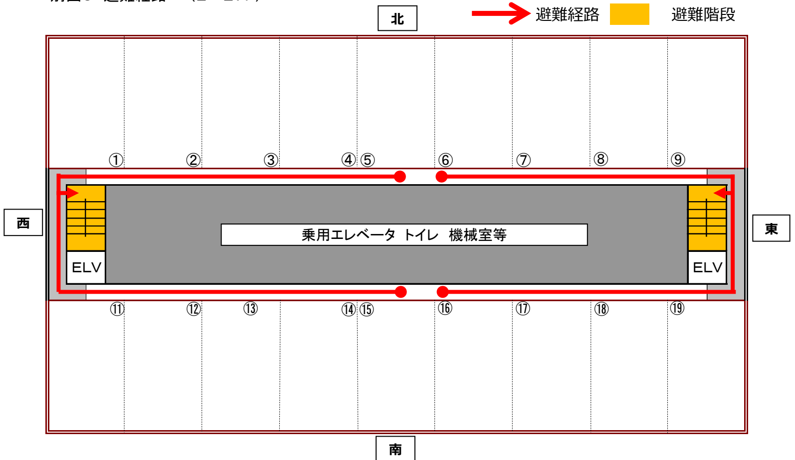
別図6 避難経路 (2~27F)
